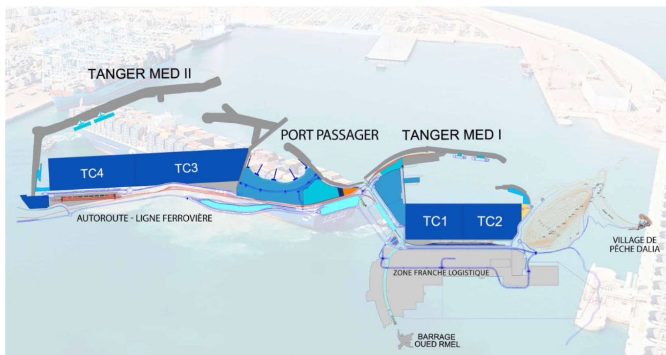
Les emplacements des terminaux sur le port de Tanger Med.
